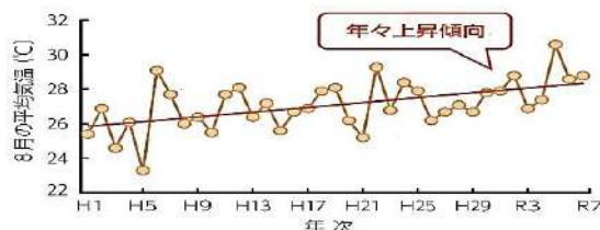
図 8月の平均気温の推移 (H1～R7 富山地方気象台)
