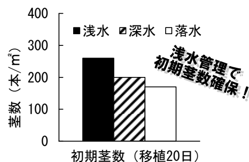
図4 初期の水管理が初期茎数に及ぼす影響 (H24 農研一部改変)
